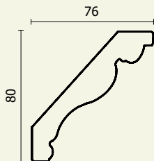
DD Карниз A1011-WG (76x80)
