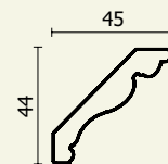
DD Карниз A1060-WG (45x44)
